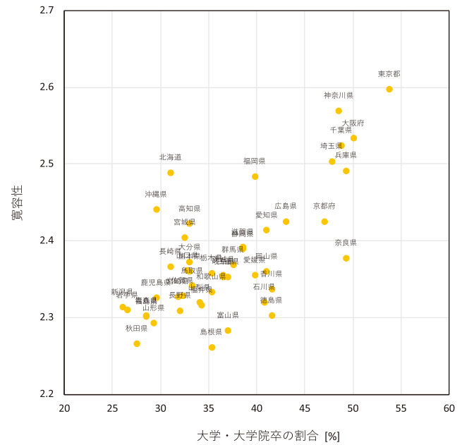
(b) 大学・大学院卒の割合（相関係数 0.692）
